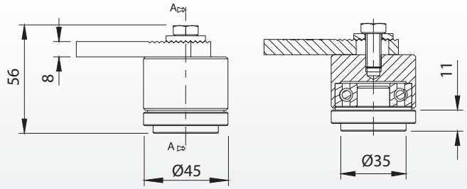
SEZ. A-A
